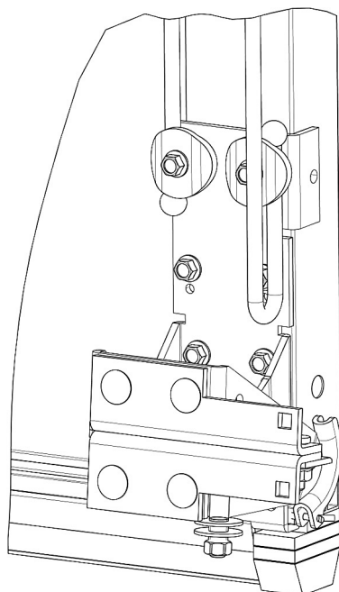
Рис. 38.2. Крепление каната
