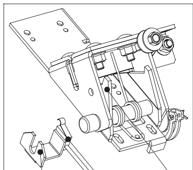
Монтажный кронштейн Микровыключатель Выступ А
