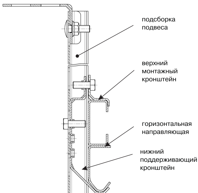
Рис.20.2. Сборка подвеса
