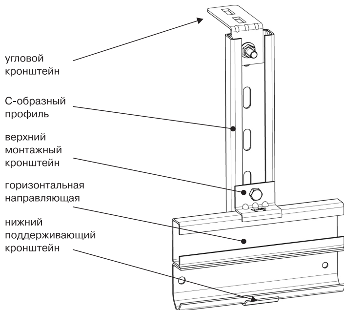
Рис.20. Подвес
