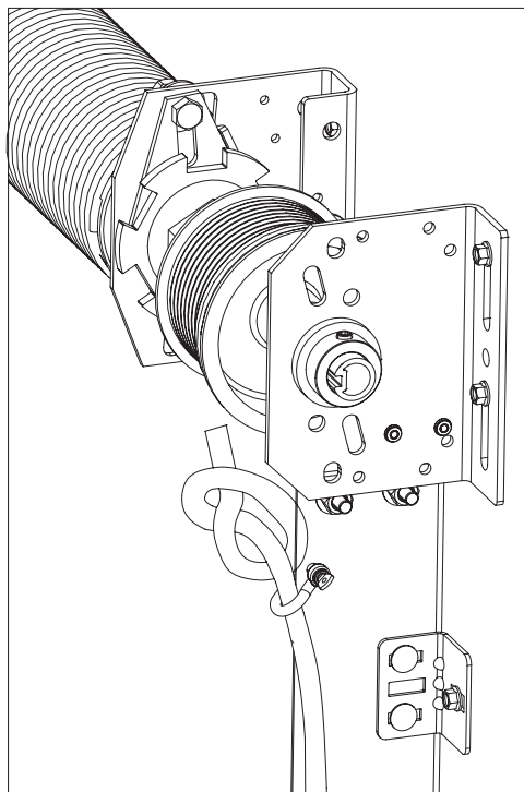
Рис. 34.1. Крепление каната к направляющей
