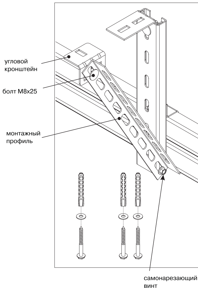
Рис.21. Установка раскоса на подвесе
