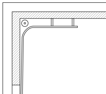
Рис. 6. Высокий монтаж с верхним расположением вала
