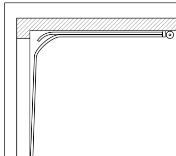
Рис. 4. Низкий монтаж
