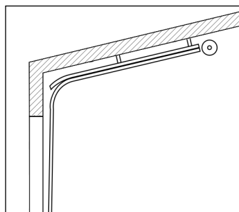
Рис. 12. Наклонный низкий монтаж
