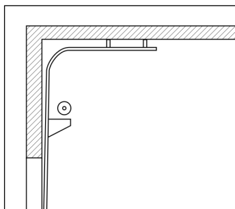
Рис. 5. Высокий монтаж с нижним расположением вала
