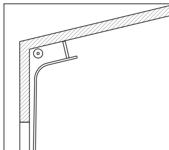
Рис. 10. Наклонный высокий монтаж с верхним расположением вала
