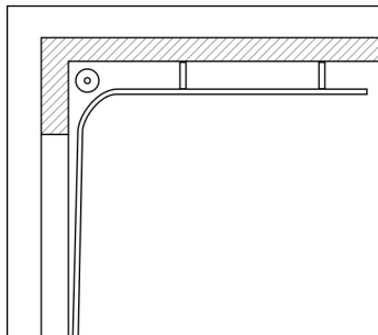
Рис. 3. Стандартный монтаж
