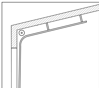
Рис. 9. Наклонный монтаж
