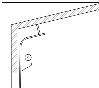
Рис. 11. Наклонный высокий монтаж с нижним расположением вала
