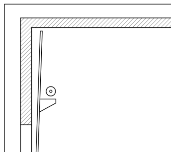
Рис. 8. Вертикальный монтаж с нижним расположением вала
